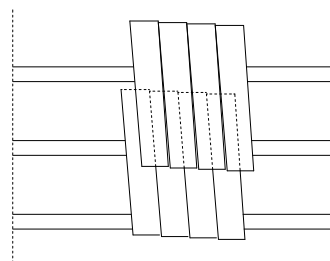
SCHEMAT UŁOŻENIA GONTU W SYSTEMIE DWUWARSTWOWYM
